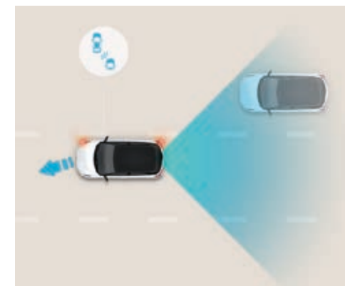
Sistema de detección de ángulo muerto (BCW). Mediante dos sensores situados en la parte inferior del parachoques trasero, el sistema te avisa de los vehículos que se acercan por la zona del ángulo muerto. Si activas el intermitente en esa dirección, el sistema emite una señal acústica (disponible en la versión Hatchback).
