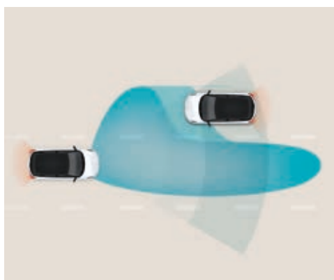
Sistema activo de luces largas (HBA). Detecta los vehículos que se aproximan y los que están en el mismo carril y cambia automáticamente a las luces cortas. Cuando no se detectan más vehículos, reactiva las luces largas para aumentar al máximo tu campo de visión.
