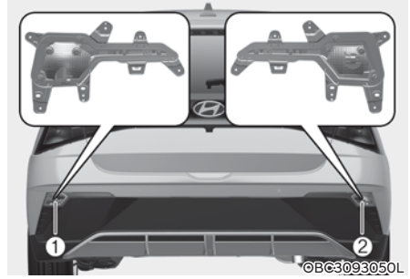
[1]: Arka Sis Lambası, [2] : Geri vites Lambası
