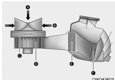
[A]: Vnější vzduch, [B]: Recirkulovaný vzduch [C]: Kabinový vzduchový filtr, [D]: Ventilátor [E]: Jádru výparníku, [F]: Jádru výměníku tepla
