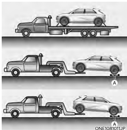
[A]: Podvalníky
