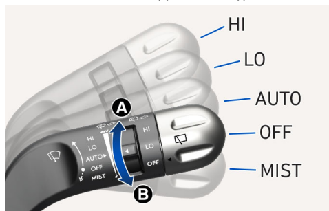
Vindusvisker/-spyler foran - Type A
