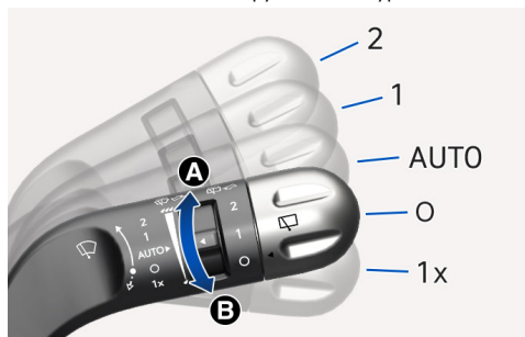
Vindusvisker/-spyler foran - Type B
