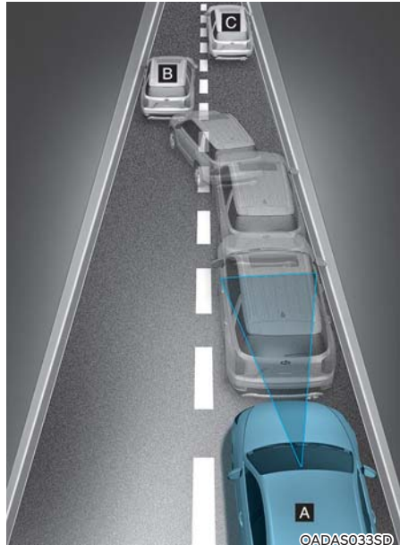
[A]: Uw voertuig, [B]: Voertuig wisselt van rijstrook, [C]: Voertuig in dezelfde rijstrook
