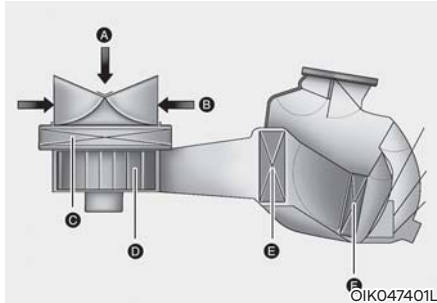
[A]: Buitenlucht, [B]: Gerecirculeerde lucht [C]: Interieurfilter, [D]: Aanjager [E]: Kachelradiateur, [F]: Verdampers
