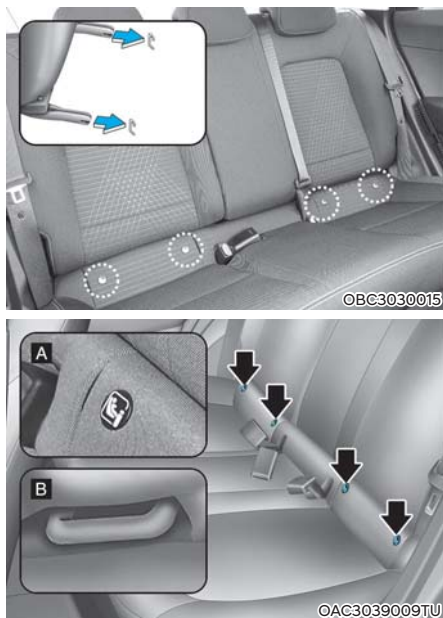
[A]: Positie-indicator ISOFIX-bevestigingspunt, [B]: ISOFIX-bevestigingspunt
